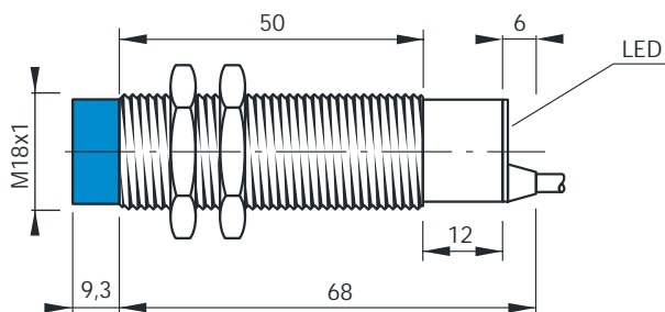
Kabelgerät / Configuration with Cable
