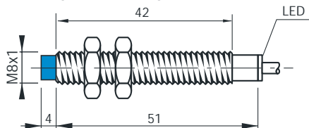
Kabelgerät / Configuration with Cable
