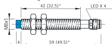
Steckergerät / Connector K1
