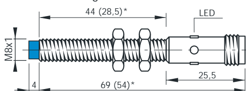
Steckergerät / Connector K
